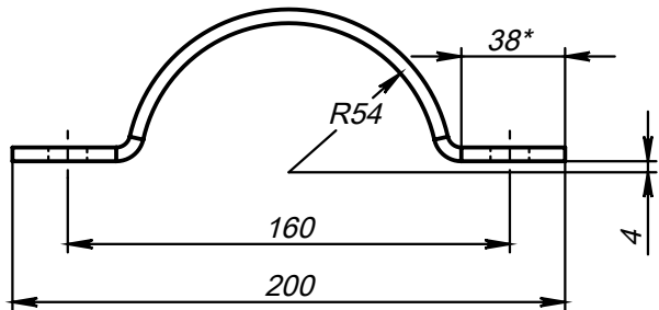
Поз.10 (Полухомут) развертка
