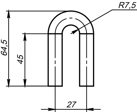
Поз.2 (Ушко) 1 : 2
