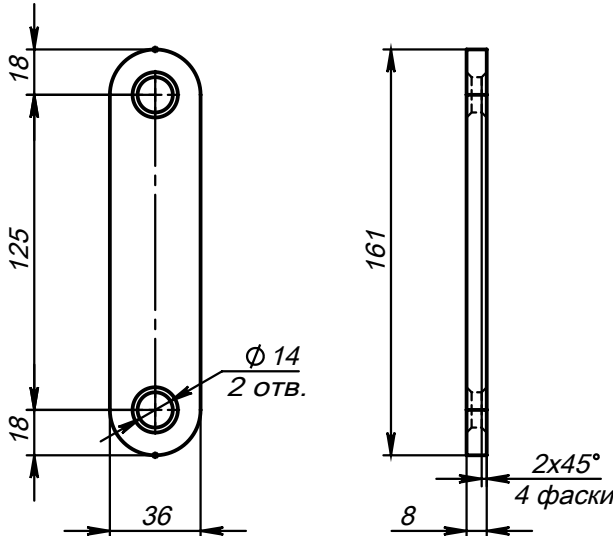
Поз.9 (Серьга)
