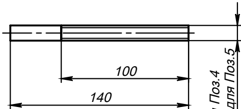
Поз.4 и Поз.5 (Шпилька)
