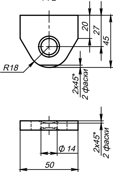
Поз.1 (Проушина) 1 : 2
