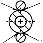
A-A (1 : 2)
